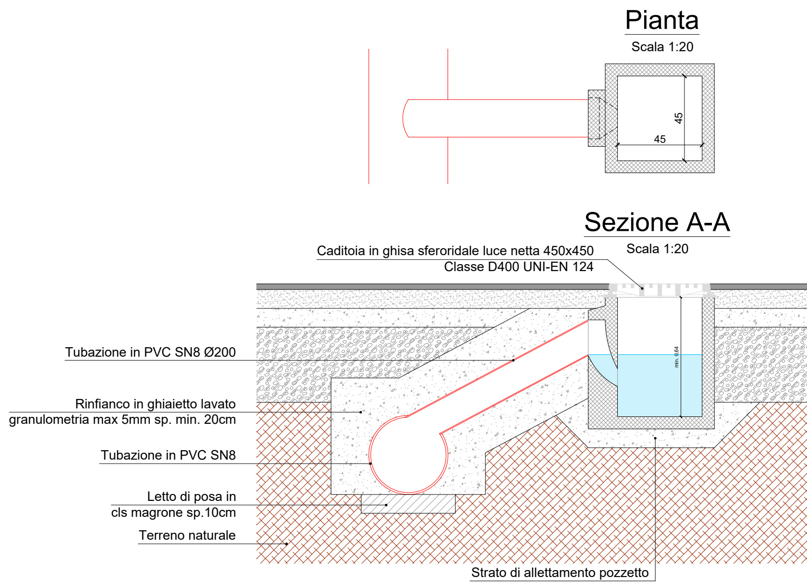
PARTICOLARE 04 - Scala 1:20 PARTICOLARE CADITOIA E COLLEGAMENTO CONDOTTA
